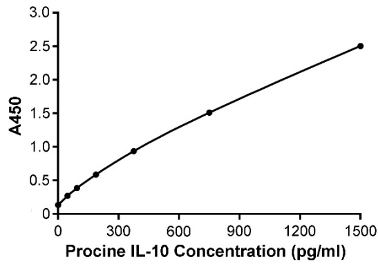
图3. Porcine IL-10 ELISA Kit的标准曲线。实测数据会因实验条件、检测仪器等的不同而存在差异，图中数据仅供参考。
